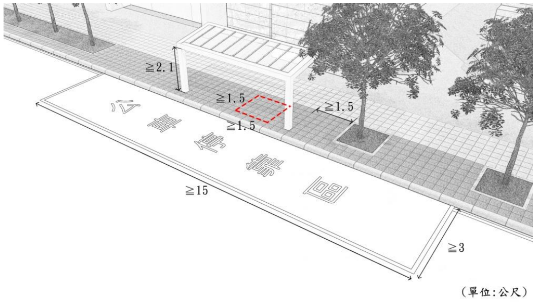
公車站臺設置參考圖
